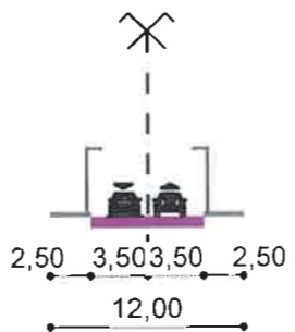
PROFIL TRANSVERSAL str.Carpati existent si mentinut
